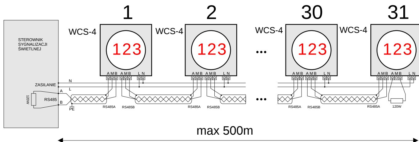
Schemat podłączenia
