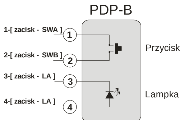
Numerzy przewodów przycisku i miejsce ich podłączenia w PDP-B
